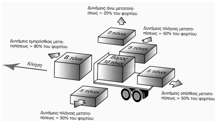
Εικ. 35 Παράδειγμα υπολογισμού Δυνάμεων Φορτίου
