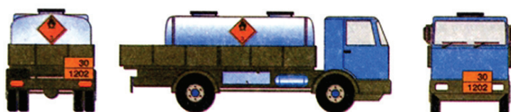
Εικ. 86 Τοποθέτηση πινακίδων αναγνώρισης υλικού και ετικετών κινδύνου σε όχημα που φέρει αποσπώμενο βυτίο με εύφλεκτα υγρά.
