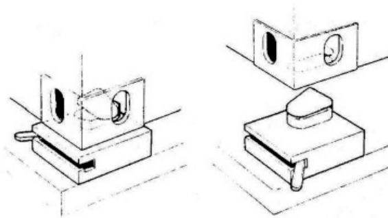
Εικ. 37 Γωνιακά σημεία κλειδώματος για ένα εμπορευματοκιβώτιο ή swap body.
